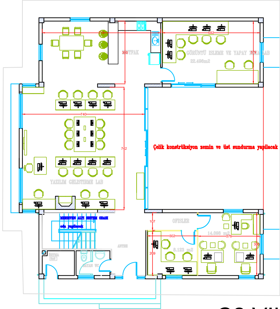
C2 VILLA Giriş kat 165m2
